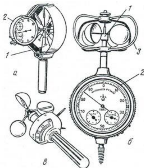
Рисунок 2 - Анемометры: а - ручной крыльчатый (вентиляционный); б - ручной чашечный; в - ручной индукционный
