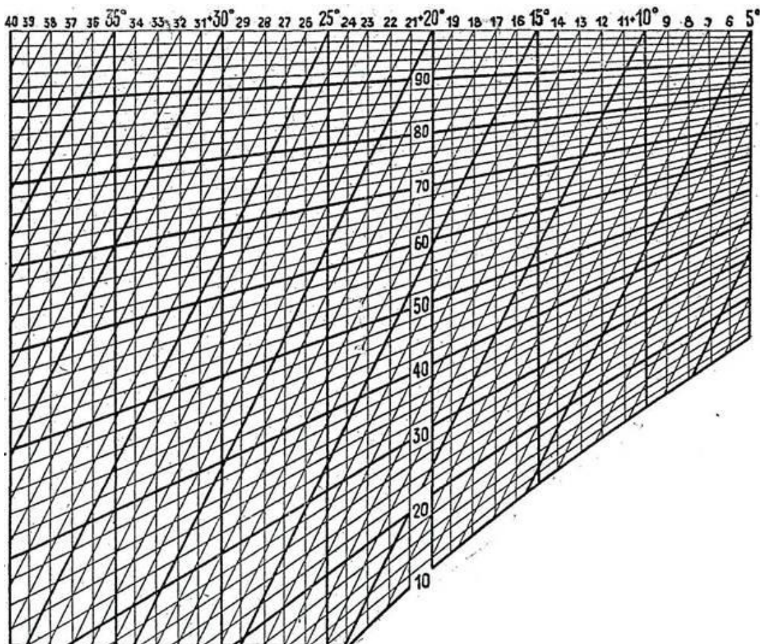
Рисунок 1 – Психрометрический график
